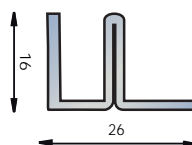
KARM PROFIL
